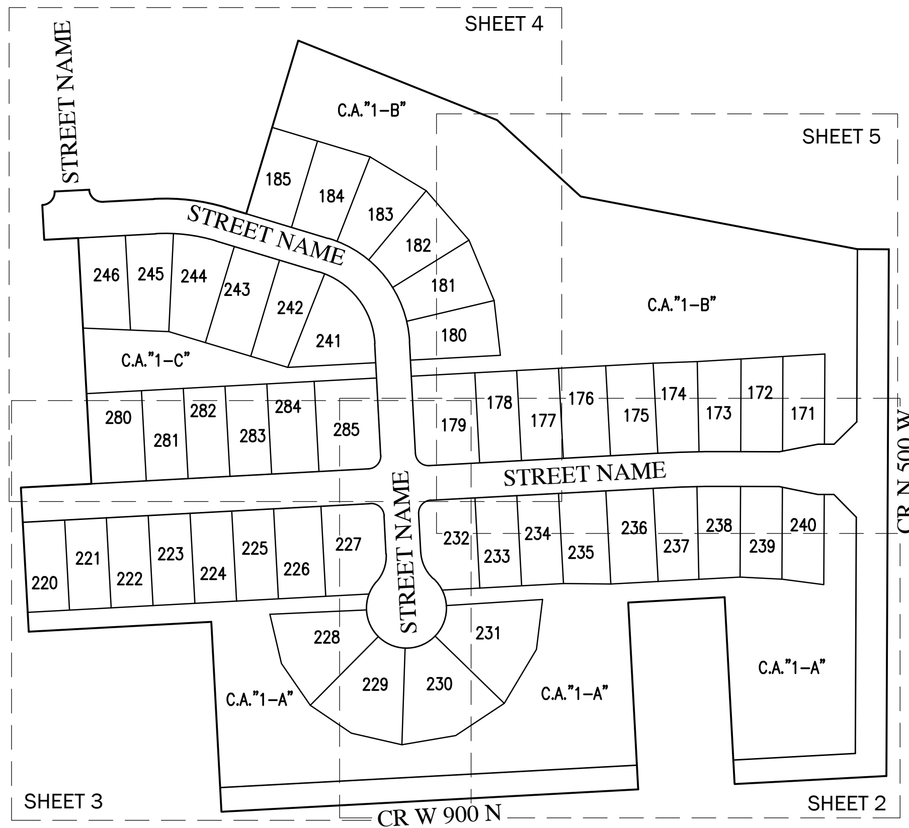
Site Map SCALE: 1" = 150'
